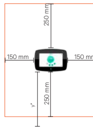
I-2.1 : Surface de montage
